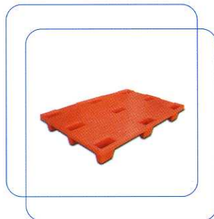
Ref. 1208 C | 9 patas Dim. Ext. 1200 x 800 x 145 Carga dinâmica até 850 kg Carga estática até 3400 kg superfície lisa
