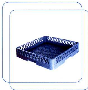
Tabuleiro rack simples ref. 9100 Dimensões exteriores: 500x500x100 mm Altura empilhada: 94 mm Abertura da rede: 9,8 mm
