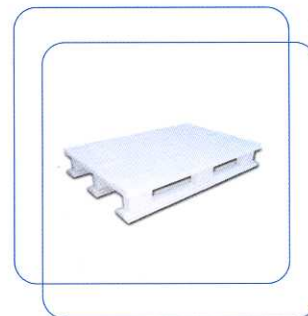
Ref. 1208 CT | 3 travessões Dim. Ext. 1200 x 800 x 170 Carga dinâmica até 1000 kg Carga estática até 4000 kg superfície lisa
